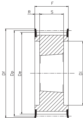
Tipo / Type 4F
