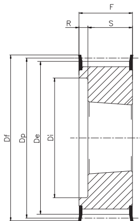
Tipo / Type 3F
