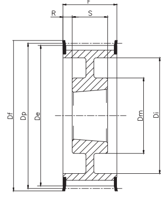
Tipo / Type 9WF
