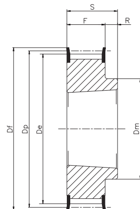
Tipo / Type 8F
