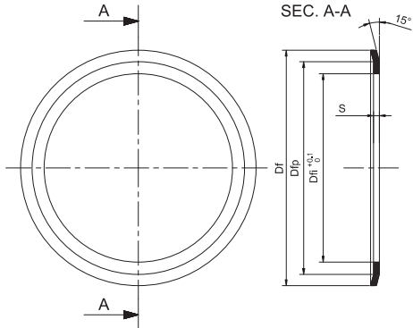
Dimensioni delle flange / Flange dimensions Bordscheiben-Abmessungen / Dimension de flasque Dimensiones de las bridas
