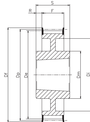
Tipo / Type 7WF
