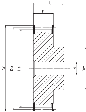
Tipo / Type 6F
