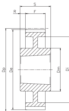
Tipo / Type 7W
