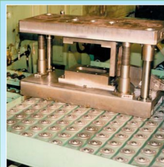
Kuličkový stůl před lisem pro rychlou výměnu tvářecích nástrojů
