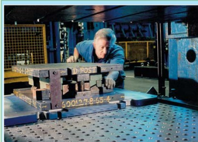
Lože lisu 600 t osazené jednotkami DL pro snadné zavedení a fixaci tvářecího nástroje
