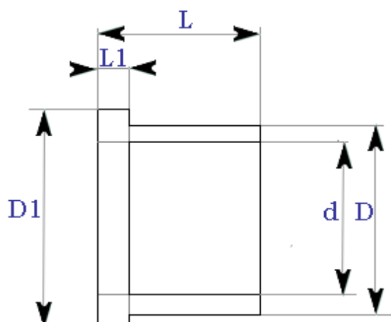
PŘÍRUBOVÁ POUZDRA
