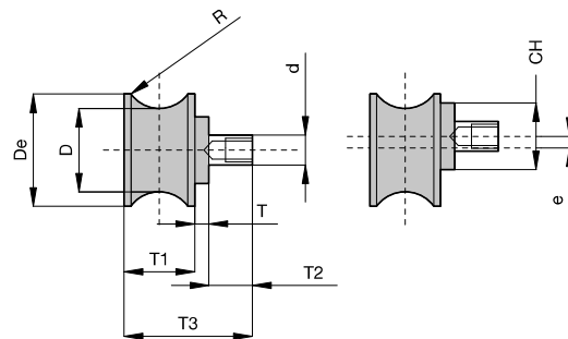
Rotella Tipo B / B type track roller
