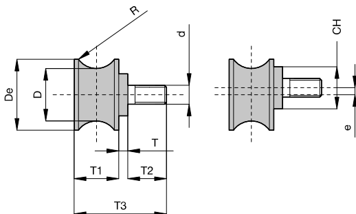
Rotella Tipo A / A type track roller
